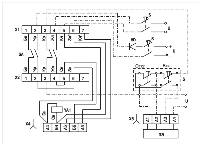
Схема соединений дополнительных сборочных единиц выключателей А3713 П, А3714 П.
